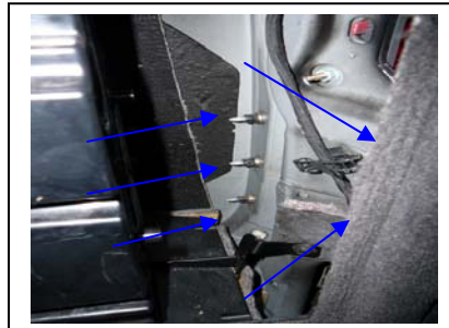
Demontage Stoßfänger Kofferraum links 5 Muttern zwei etwas versteckt Richtung Kofferraumklappe
