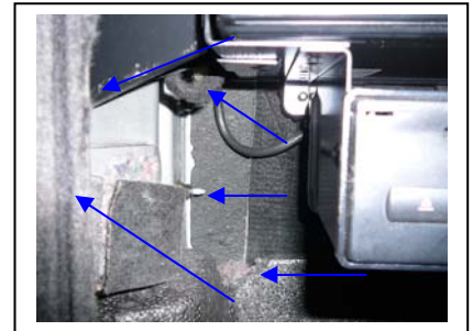
Demontage Stoßfänger Kofferraum rechts 5 Muttern zwei etwas versteckt Richtung Kofferraumklappe
